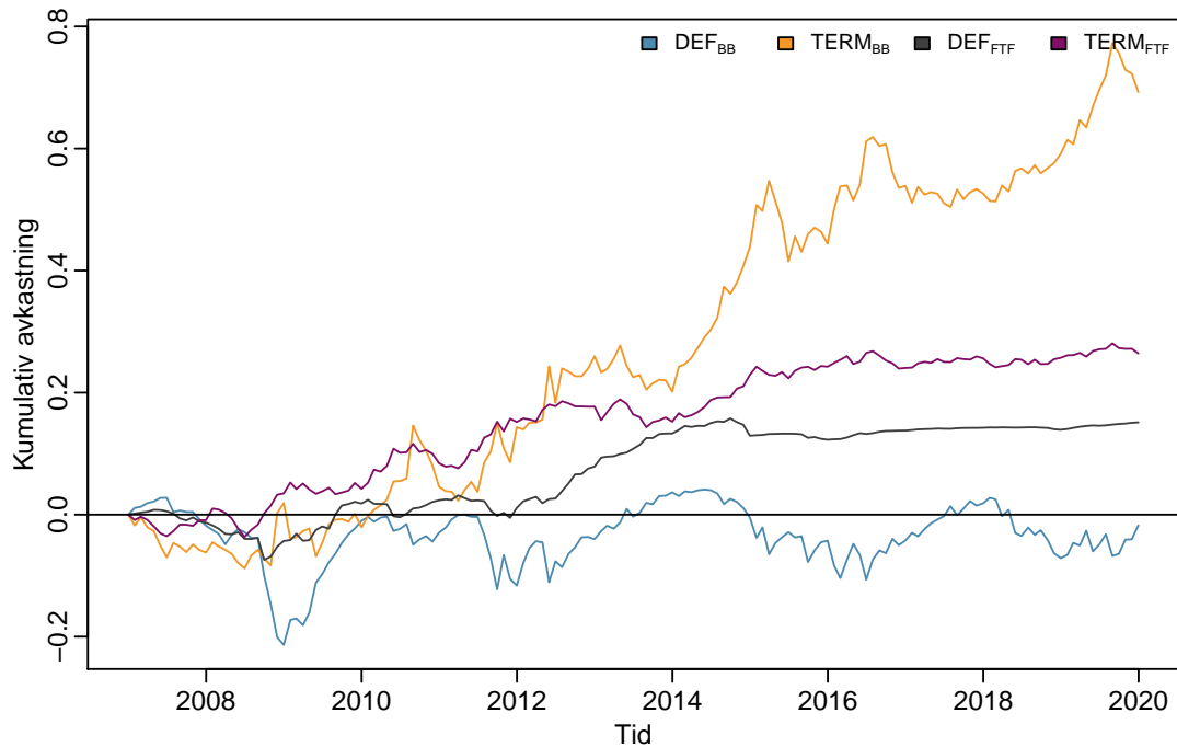
Figur C.6: Rentefaktorer
