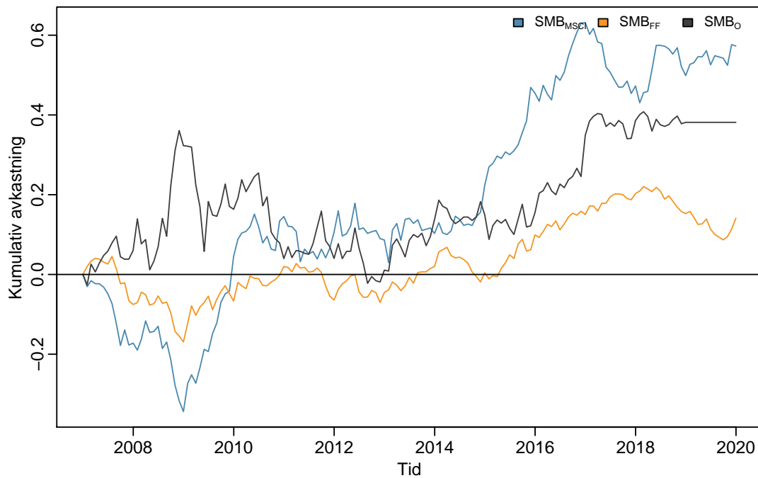
Figur C.4: SMB-faktorer
