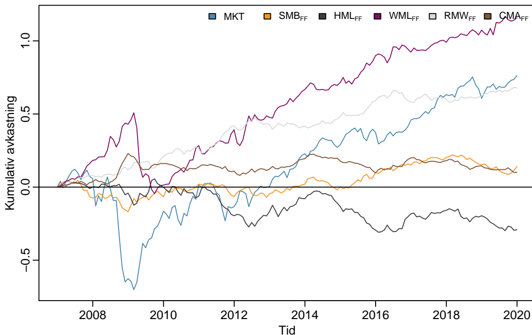
Figur C.2: Europa-faktorer
