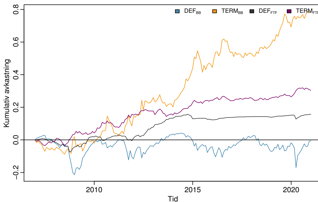
Figur C.6: Rentefaktorer
