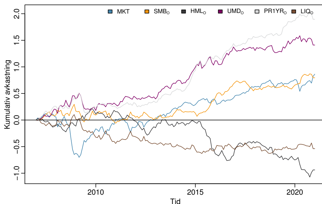
Figur C.3: Norge-faktorer
